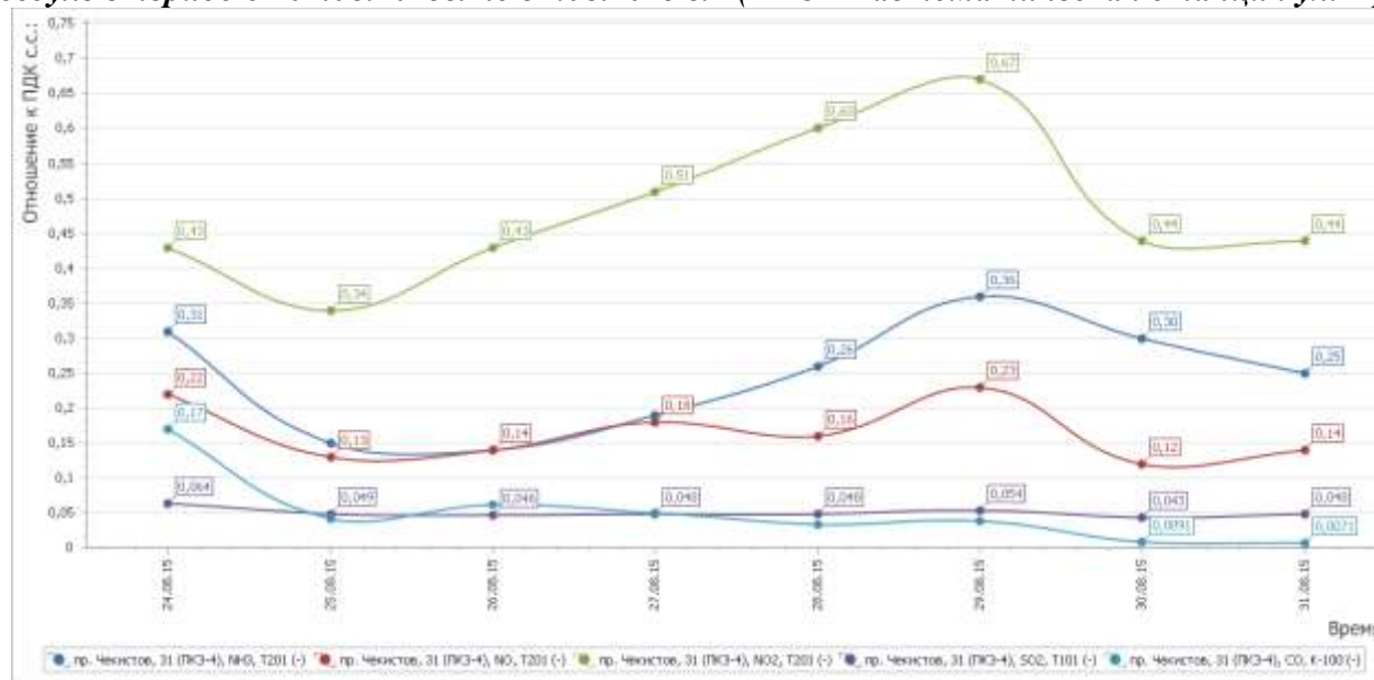
Рисунок 6 - График среднесуточных значений концентраций загрязняющих веществ (в долях ПДК) в атмосферном воздухе в период с 01.08.2015г. по 31.08.2015 г. (ПКЗ 4 - автоматическая станция ул. Проспект Чекистов)
