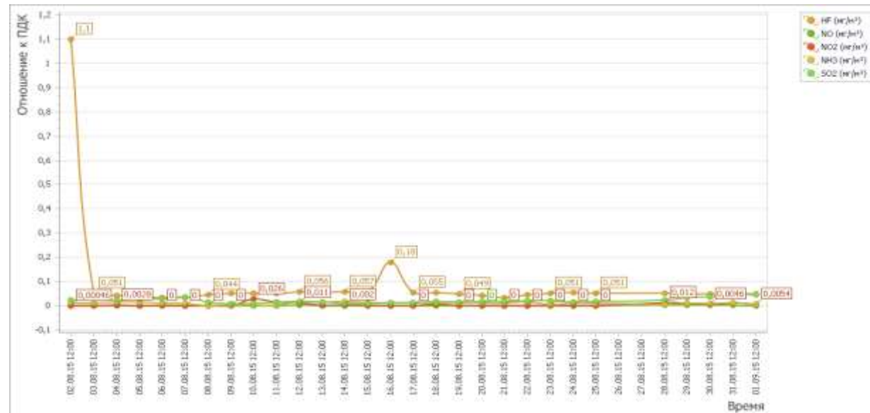
Рисунок 2 – График среднесуточных значений концентраций загрязняющих веществ в атмосферном воздухе (в долях ПДК) в период с 01.08.2015г. по 31.08.2015 г. (автоматическая станция п. Мирный)
