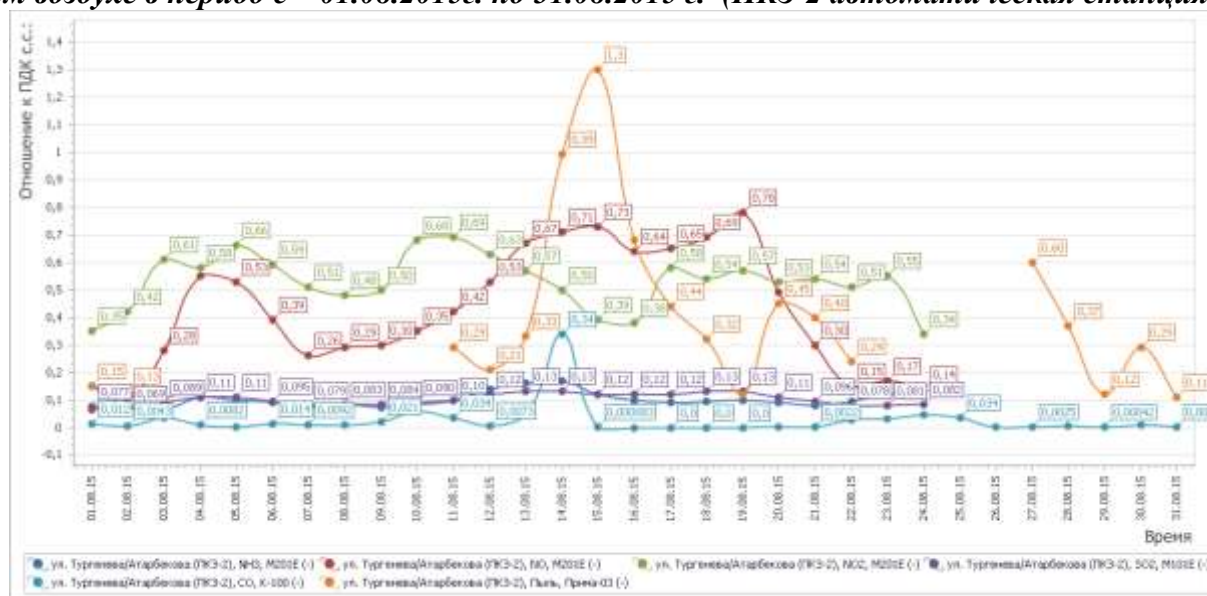
Рисунок 4 - График среднесуточных значений концентраций загрязняющих веществ (в долях ПДК) в атмосферном воздухе в период с 01.08.2015г. по 31.08.2015 г. (ПКЗ-2 автоматическая станция ул.Атарбекова)
