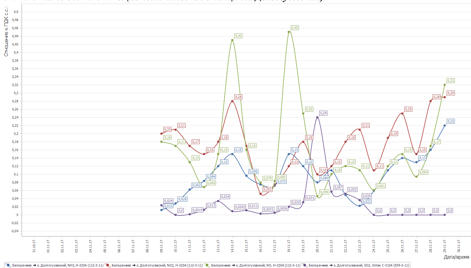
Рисунок 1- График среднесуточных значений концентраций загрязняющих веществ (в долях ПДК) в атмосферном воздухе в период с 01.11.2017г. по 30.11.2017 г. (автоматическая станция х. Долгогусевский)
