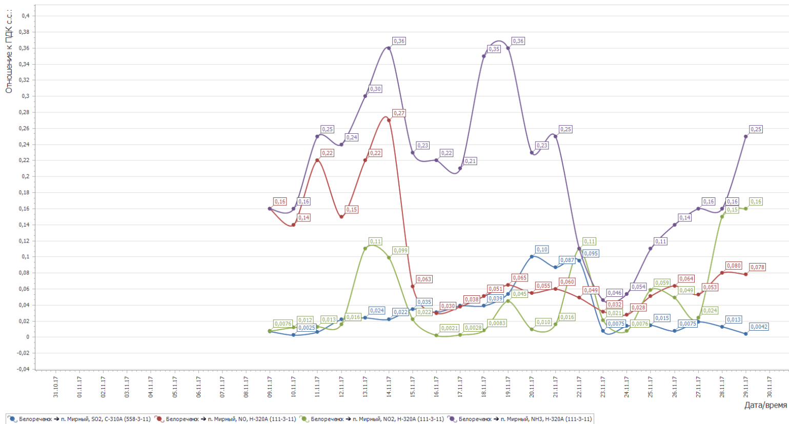
Рисунок 2- График среднесуточных значений концентраций загрязняющих веществ (в долях ПДК) в атмосферном воздухе в период с 01.11.2017г. по 30.11.2017 г. (автоматическая станция п. Мирный)
