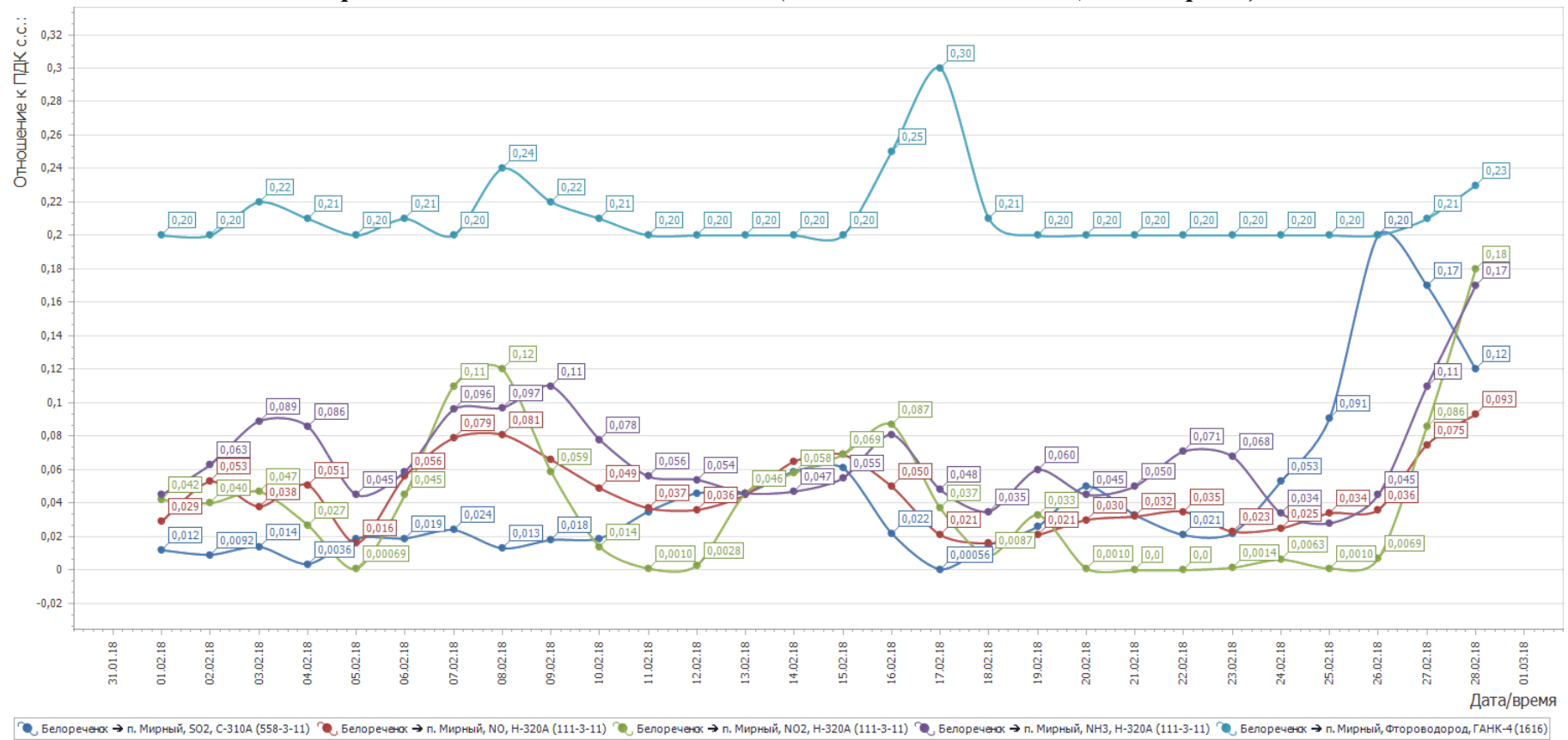
Рисунок 2- График среднесуточных значений концентраций загрязняющих веществ (в долях ПДК) в атмосферном воздухе в период с 01.02.2018г. по 28.02.2018 г. (автоматическая станция п. Мирный)
