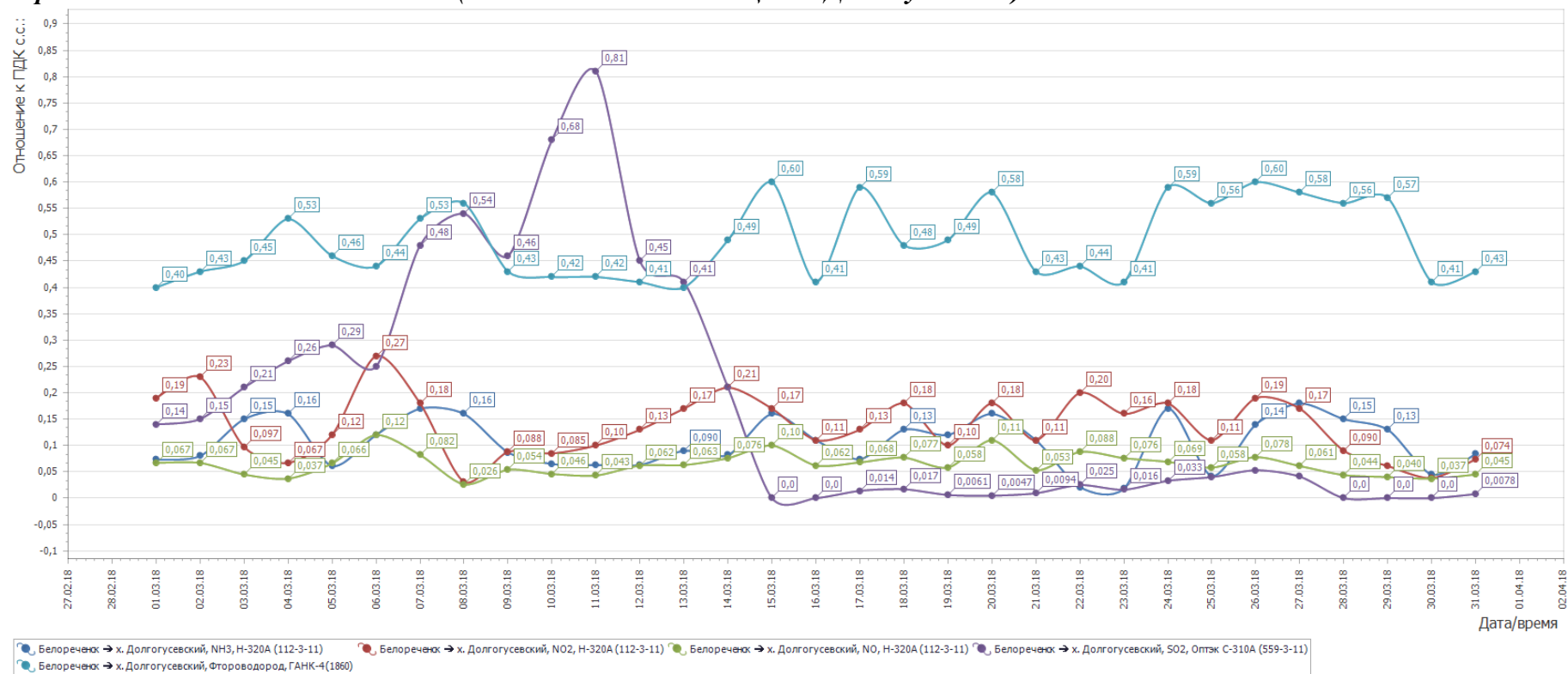
Рисунок 1- График среднихсуточных значений концентраций загрязняющих веществ (в долях ПДК) в атмосферном воздухе в период с 01.03.2018г. по 31.03.2018 г. (автоматическая станция х. Долгогусевский)
