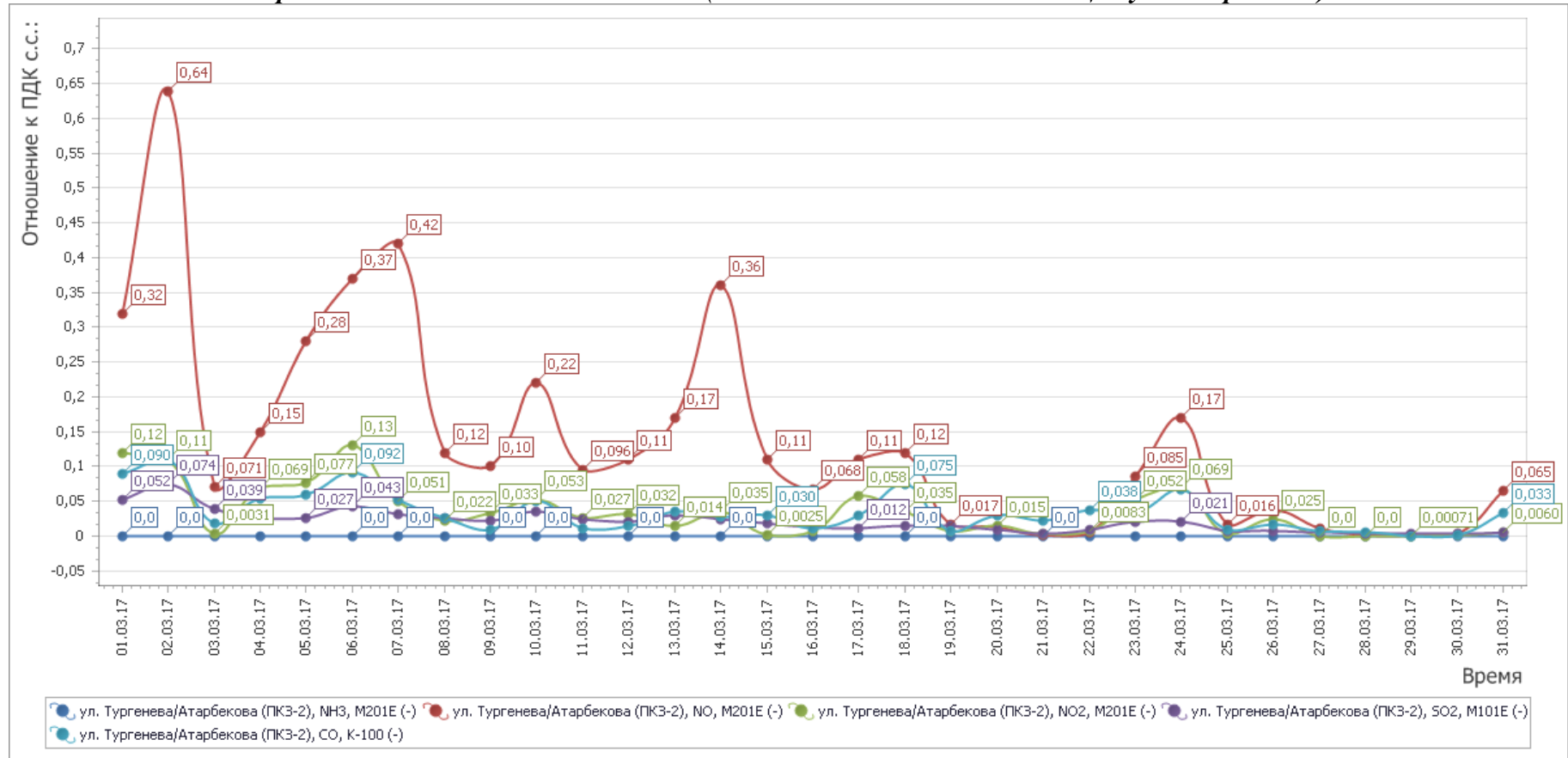
Рисунок 4 - График среднесуточных значений концентраций загрязняющих веществ (в долях ПДК) в атмосферном воздухе в период с 01.03.2017г. по 31.03.2017 г. (ПКЗ-2 автоматическая станция ул. Атарбекова)
