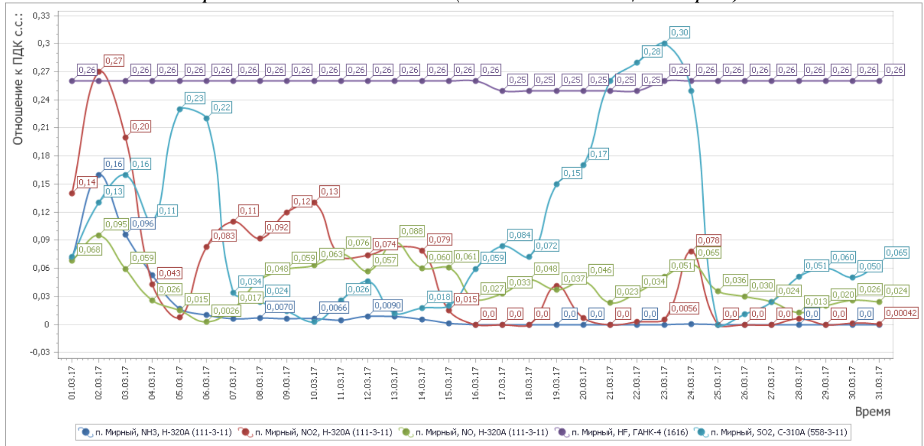
Рисунок 2- График среднесуточных значений концентраций загрязняющих веществ (в долях ПДК) в атмосферном воздухе в период с 01.03.2017г. по 31.03.2017 г. (автоматическая станция п. Мирный)
