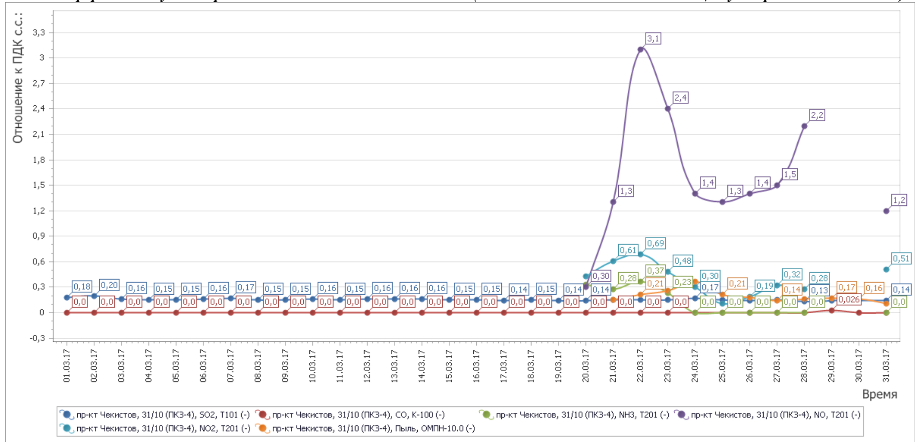
Рисунок 6 - График среднесуточных значений концентраций загрязняющих веществ (в долях ПДК) в атмосферном воздухе в период с 01.03.2017г. по 31.03.2017 г. (ПКЗ 4 - автоматическая станция ул. Проспект Чекистов)
