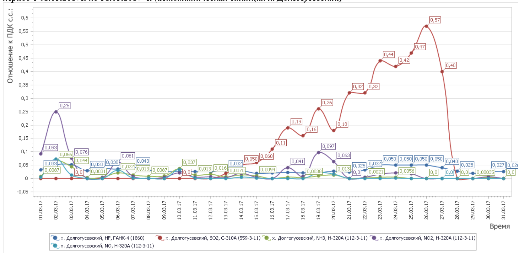
Рисунок 1- График среднесуточных значений концентраций загрязняющих веществ (в долях ПДК) в атмосферном воздухе в период с 01.03.2017г. по 31.03.2017 г. (автоматическая станция х. Долгогусевский)
