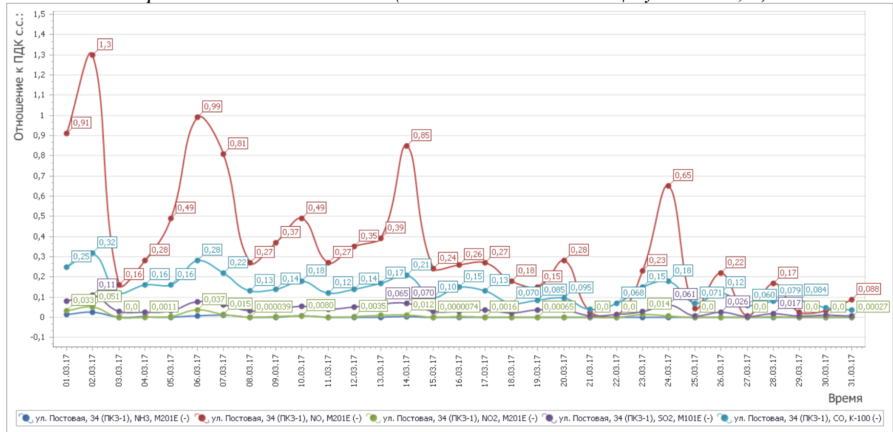
Рисунок 3- График среднесуточных значений концентраций загрязняющих веществ (в долях ПДК) в атмосферном воздухе в период с 01.03.2017г. по 31.03.2017 г. (ПКЗ-1 - автоматическая станция ул. Постовая, 34)
