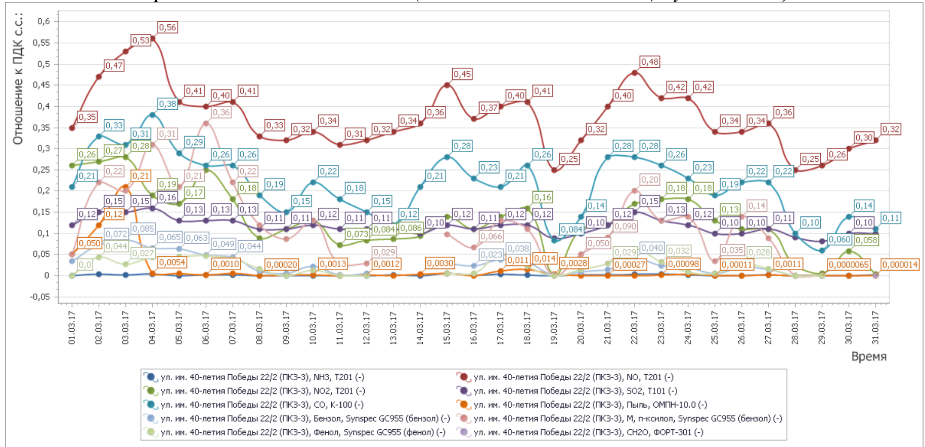
Рисунок 5 - График среднесуточных значений концентраций загрязняющих веществ (в долях ПДК) в атмосферном воздухе в период с 01.03.2017г. по 31.03.2017 г. (ПКЗ-3 - автоматическая станция ул. Московская)
