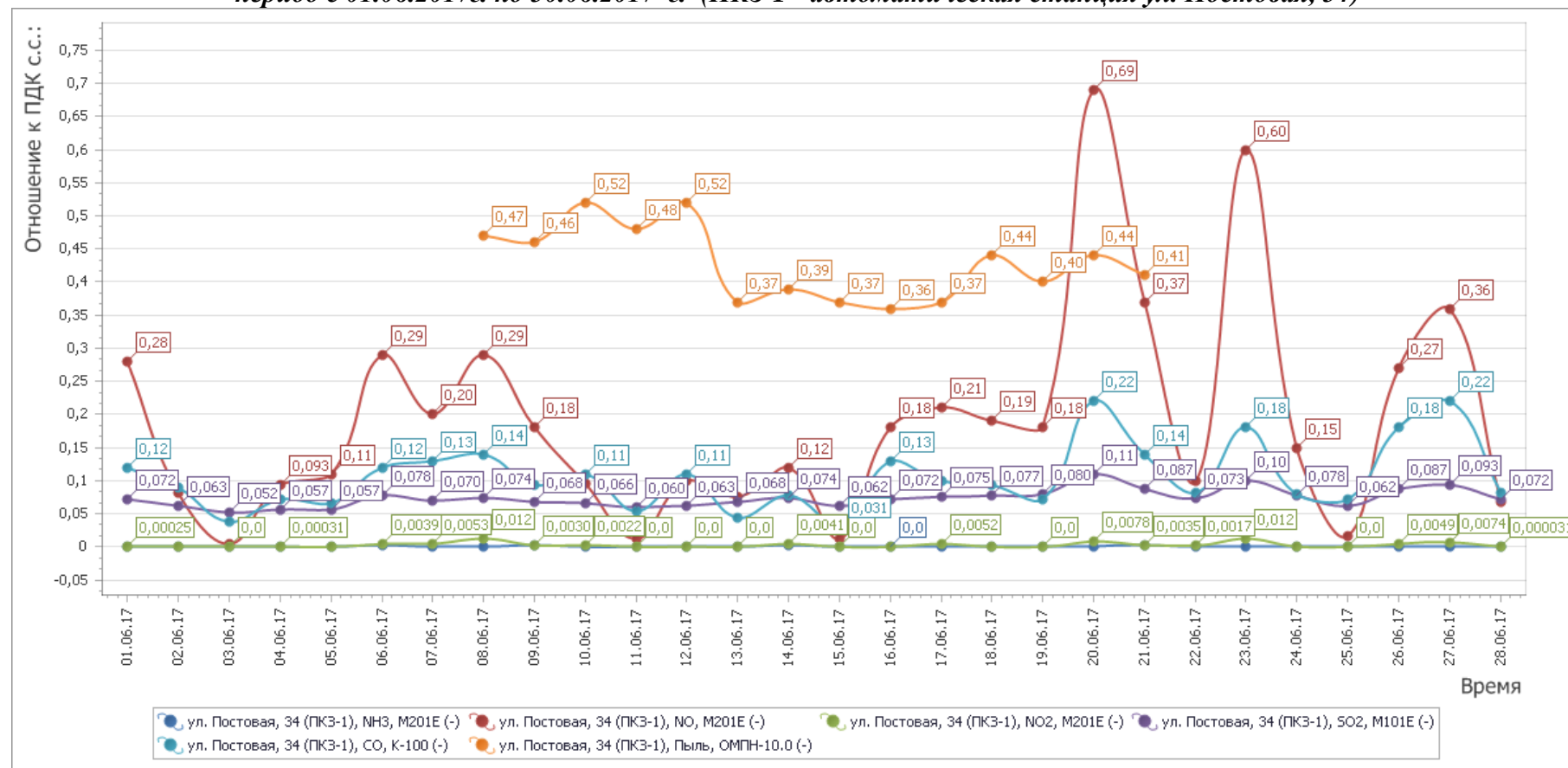
Рисунок 3- График среднесуточных значений концентраций загрязняющих веществ (в долях ПДК) в атмосферном воздухе в период с 01.06.2017г. по 30.06.2017 г. (ПКЗ-1 - автоматическая станция ул. Постовая, 34)
