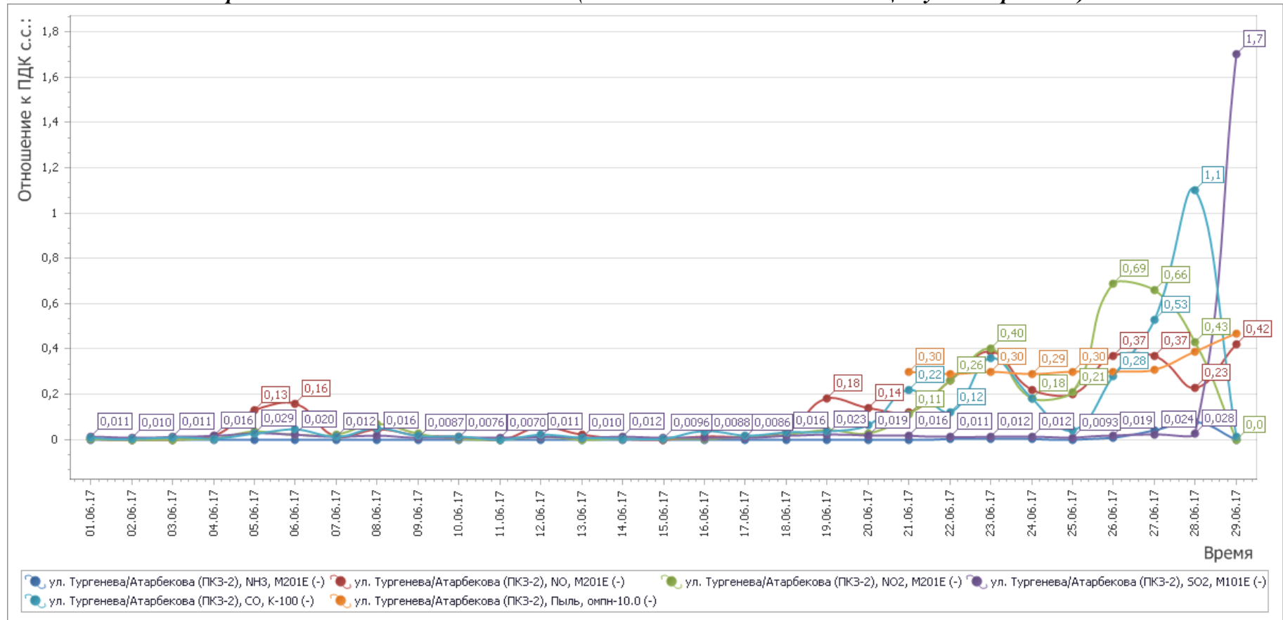
Рисунок 4 - График среднесуточных значений концентраций загрязняющих веществ (в долях ПДК) в атмосферном воздухе в период с 01.06.2017г. по 30.06.2017 г. (ПКЗ-2 автоматическая станция ул. Атарбекова)
