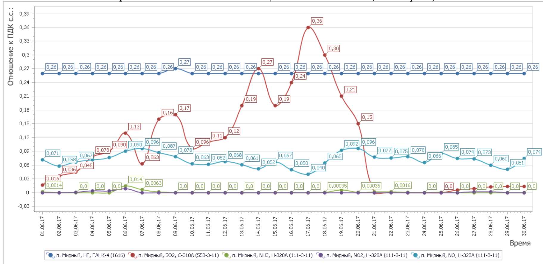
Рисунок 2- График среднесуточных значений концентраций загрязняющих веществ (в долях ПДК) в атмосферном воздухе в период с 01.06.2017г. по 30.06.2017 г. (автоматическая станция п. Мирный)
