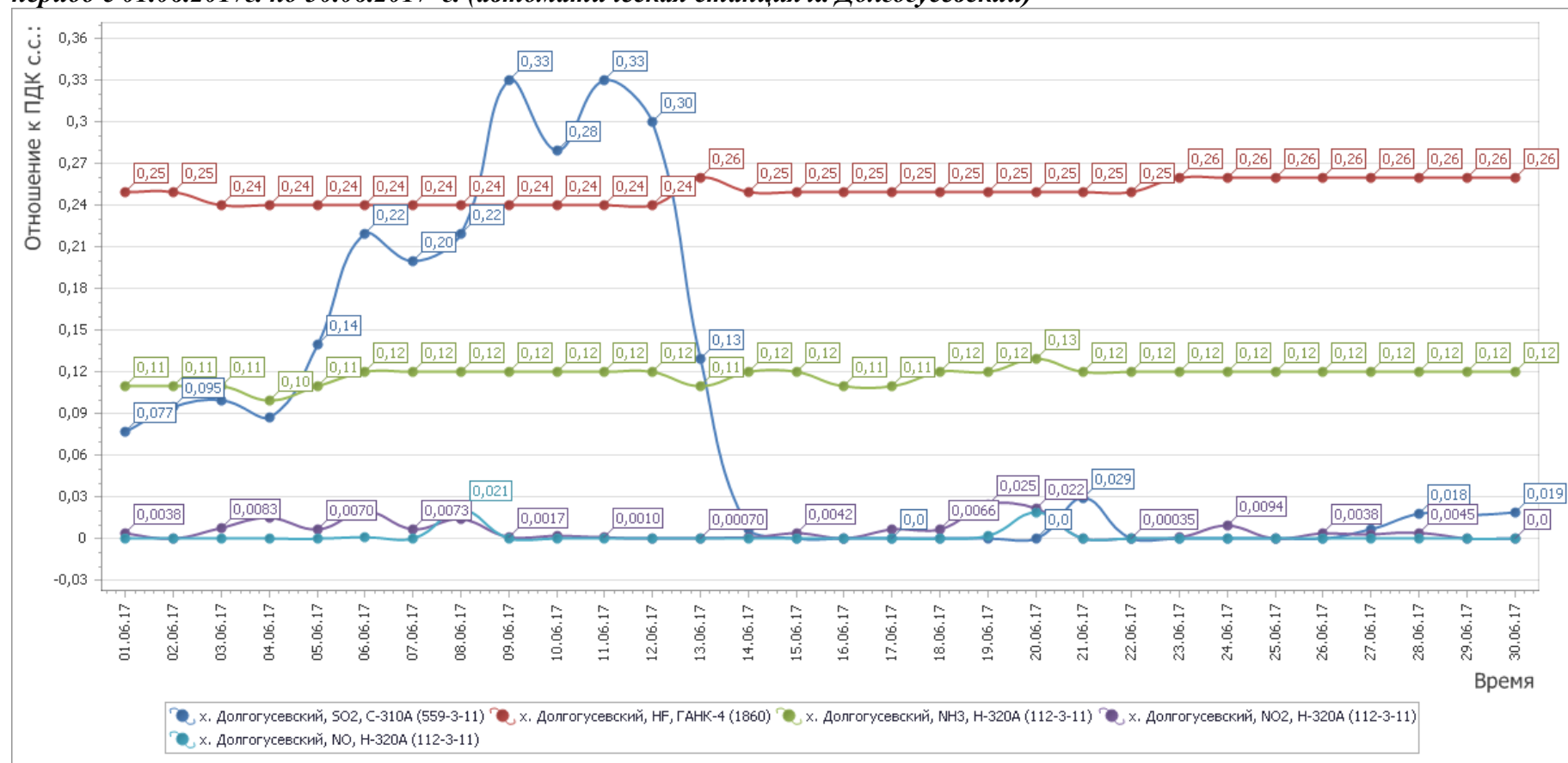
Рисунок 1- График среднесуточных значений концентраций загрязняющих веществ (в долях ПДК) в атмосферном воздухе в период с 01.06.2017г. по 30.06.2017 г. (автоматическая станция х. Долгогусевский)
