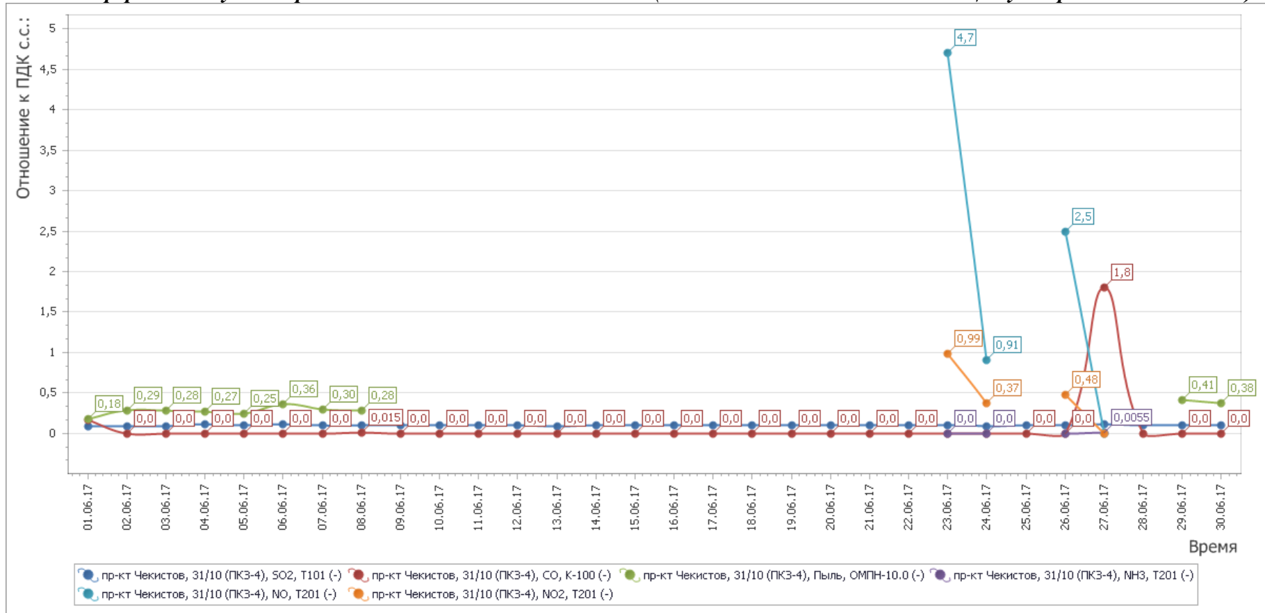
Рисунок 6 - График среднесуточных значений концентраций загрязняющих веществ (в долях ПДК) в атмосферном воздухе в период с 01.06.2017г. по 30.06.2017 г. (ПКЗ 4 - автоматическая станция ул. Проспект Чекистов)
