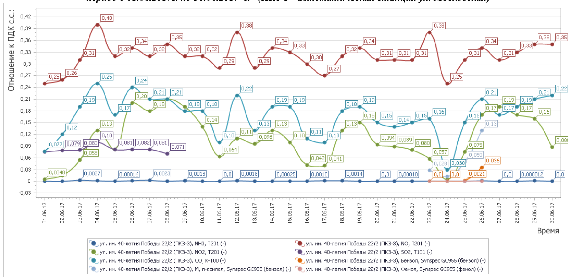
Рисунок 5 - График среднесуточных значений концентраций загрязняющих веществ (в долях ПДК) в атмосферном воздухе в период с 01.06.2017г. по 30.06.2017 г. (ПКЗ-3 - автоматическая станция ул. Московская)
