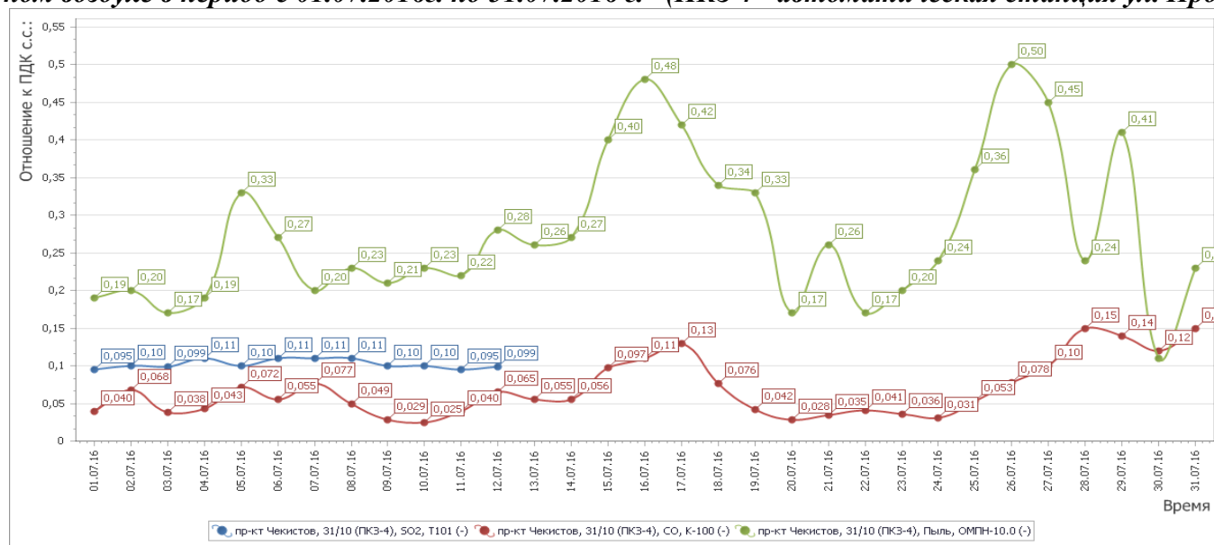
Рисунок 6 - График среднесуточных значений концентраций загрязняющих веществ (в долях ПДК) в атмосферном воздухе в период с 01.07.2016г. по 31.07.2016 г. (ПКЗ 4 - автоматическая станция ул. Проспект Чекистов)
