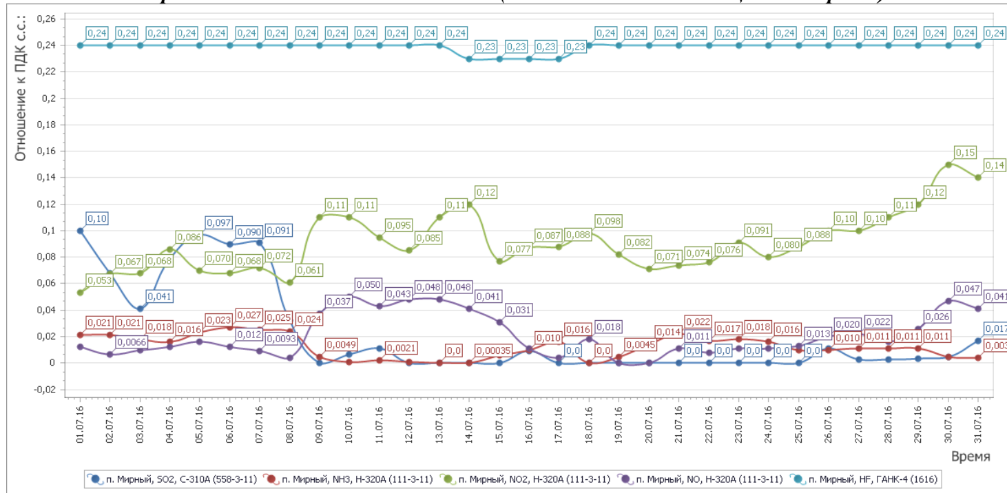
Рисунок 2- График среднесуточных значений концентраций загрязняющих веществ (в долях ПДК) в атмосферном воздухе в период с 01.07.2016г. по 31.07.2016 г. (автоматическая станция п. Мирный)
