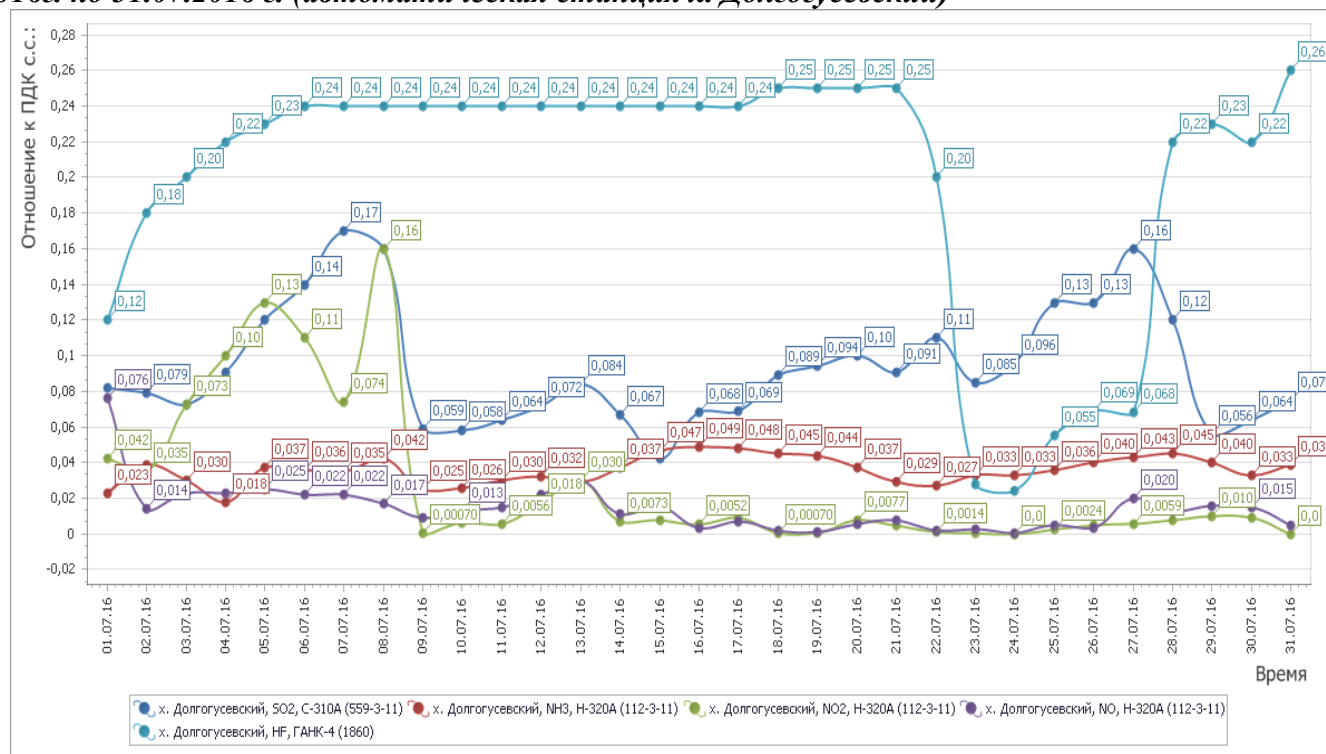
Рисунок 1- График среднесуточных значений концентраций загрязняющих веществ (в долях ПДК ) в атмосферном воздухе в период с 01.07.2016г. по 31.07.2016 г. (автоматическая станция х. Долгогусевский)
