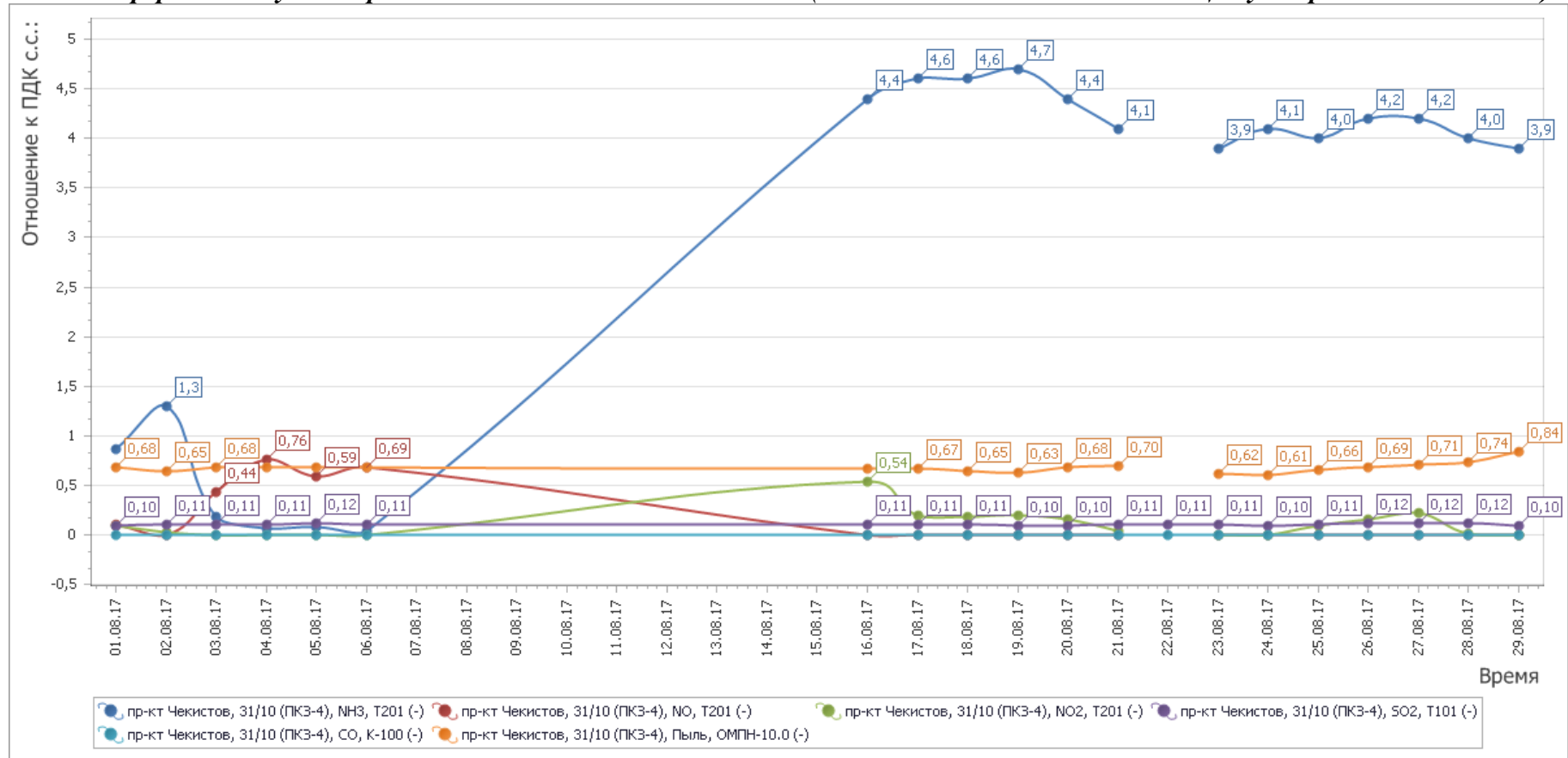
Рисунок 6 - График среднесуточных значений концентраций загрязняющих веществ (в долях ПДК) в атмосферном воздухе в период с 01.08.2017г. по 31.08.2017 г. (ПКЗ 4 - автоматическая станция ул. Проспект Чекистов)
